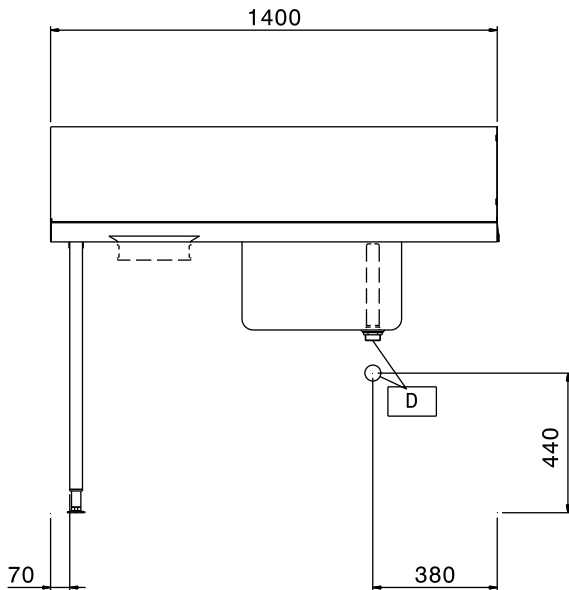
Front aanzicht
